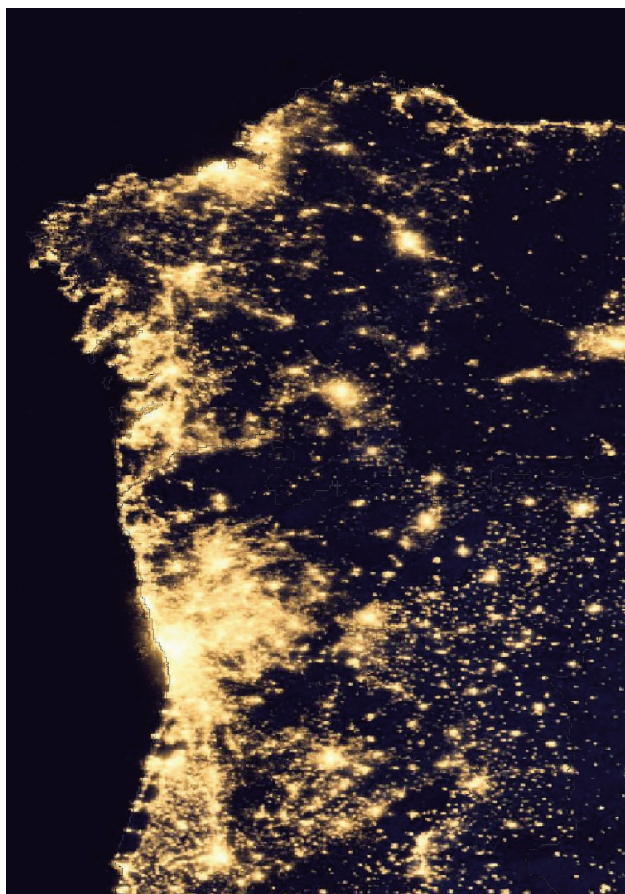
Emisións de luz cara ao ceo en Galiza e na rexión norte de Portugal. Earth at Night 2012, SUOMI-NPP VIIRS via NASA Earth Observatory, http://npp.gsfc.nasa.gov/
